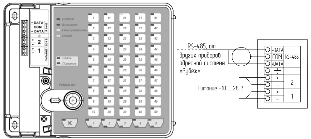
Рисунок 1 - Внешний вид и схема подключения прибора
